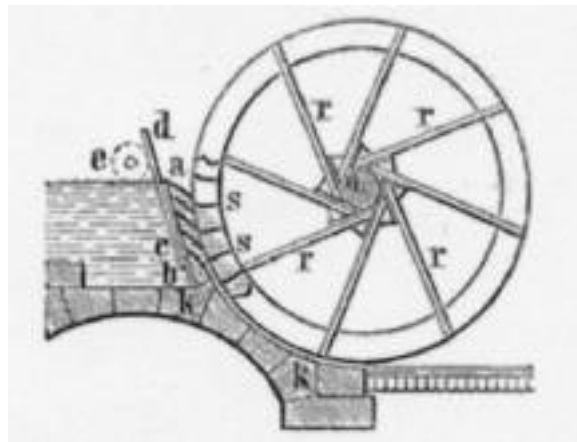
Mittelschlächtiges Wasserrad
